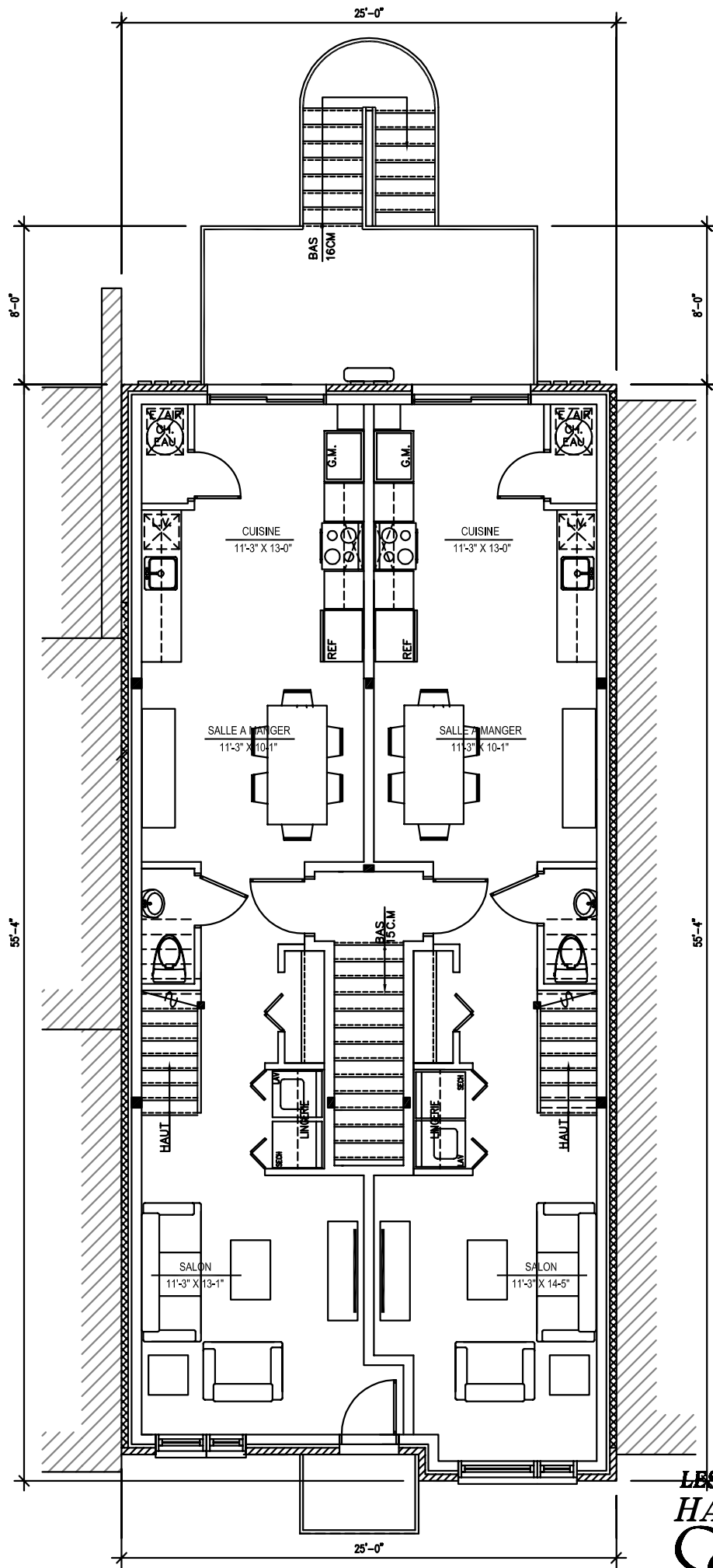
PLAN DU 2eme ETAGE
