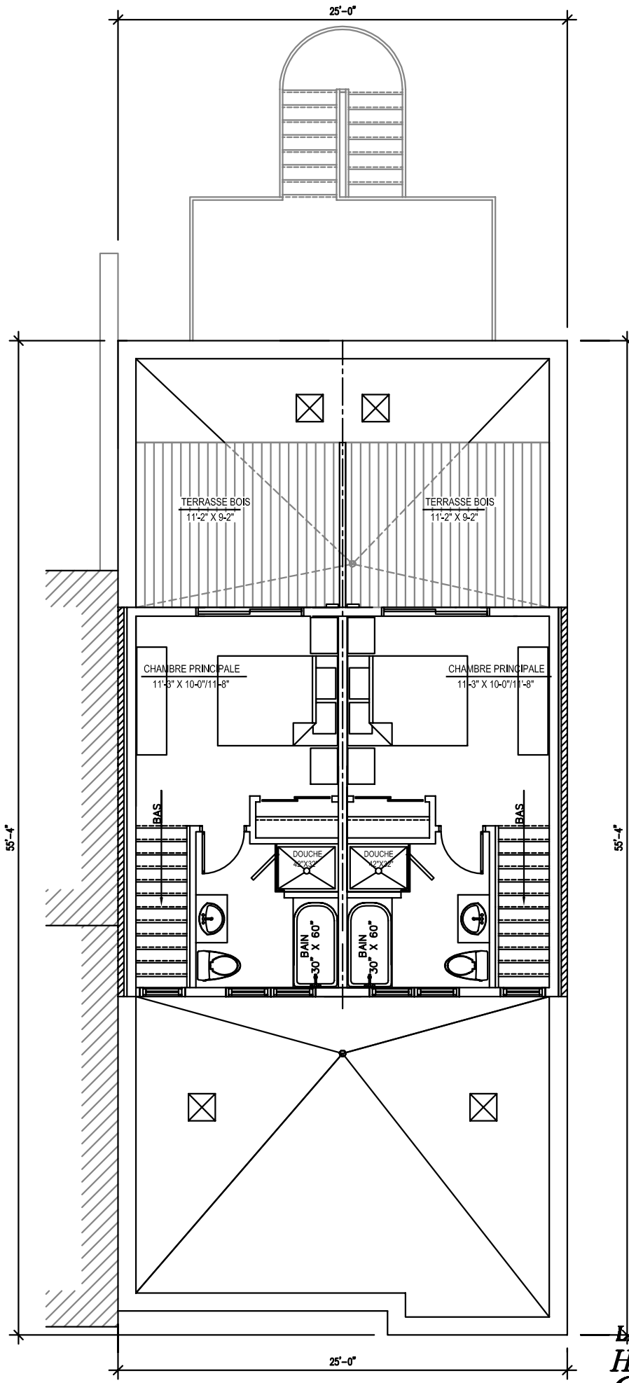
PLAN DE LA MEZZANINE / SURHAUTEUR
