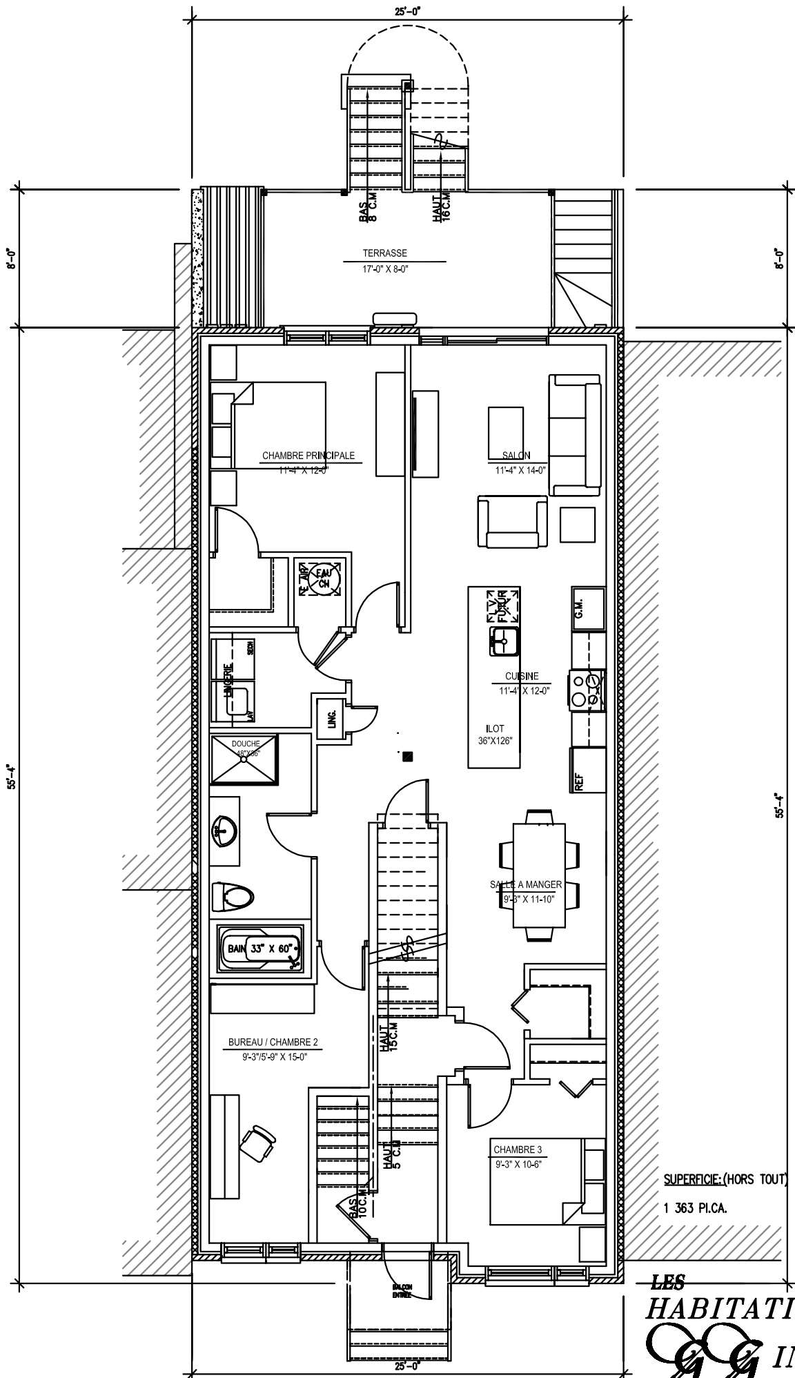
PLAN DE REZ-DE-CHAUSSEE
